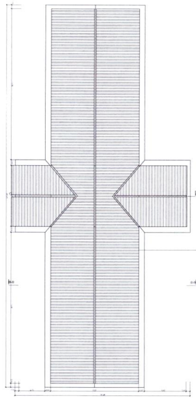
Toiture
